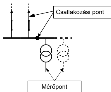
3.1./2 Egyirányú ellátás felfűzéssel (közcsélú kábelhálózat)
