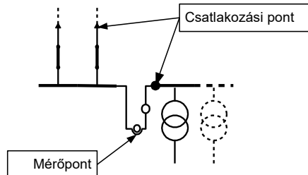
3.2./2 Mérés középfeszültségen (közcsélú kábelhálózat)
